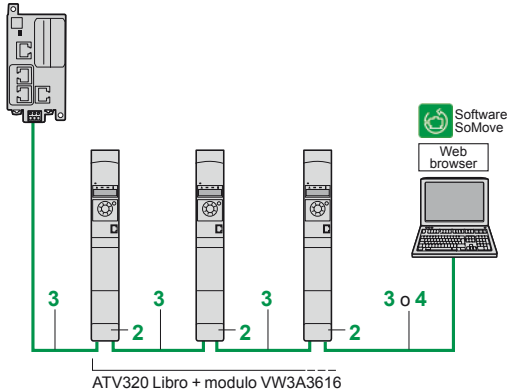
Esempio di collegamento su una rete EtherNet/IP
